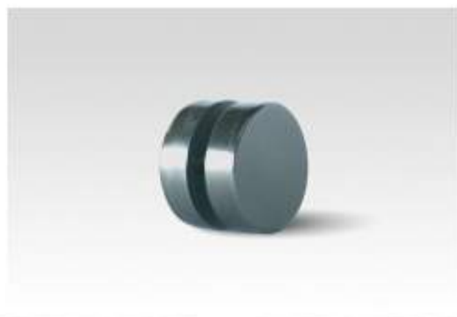
Tirador chato de Aluminio: 30mm, de diámetro, espesor 8mm.
